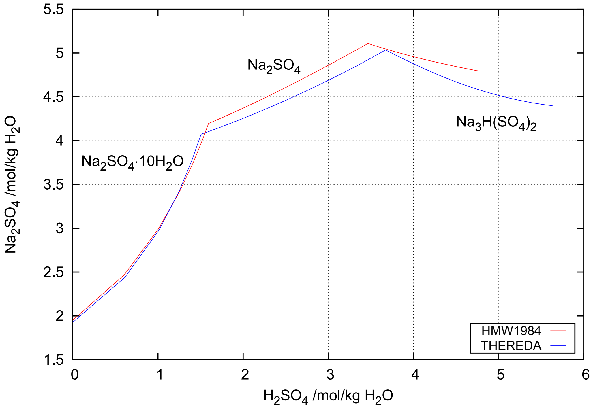
System \text{H}_2\text{SO}_4\text{-Na}_2\text{SO}_4\text{-H}_2\text{O} at T=298.15\text{ K}
