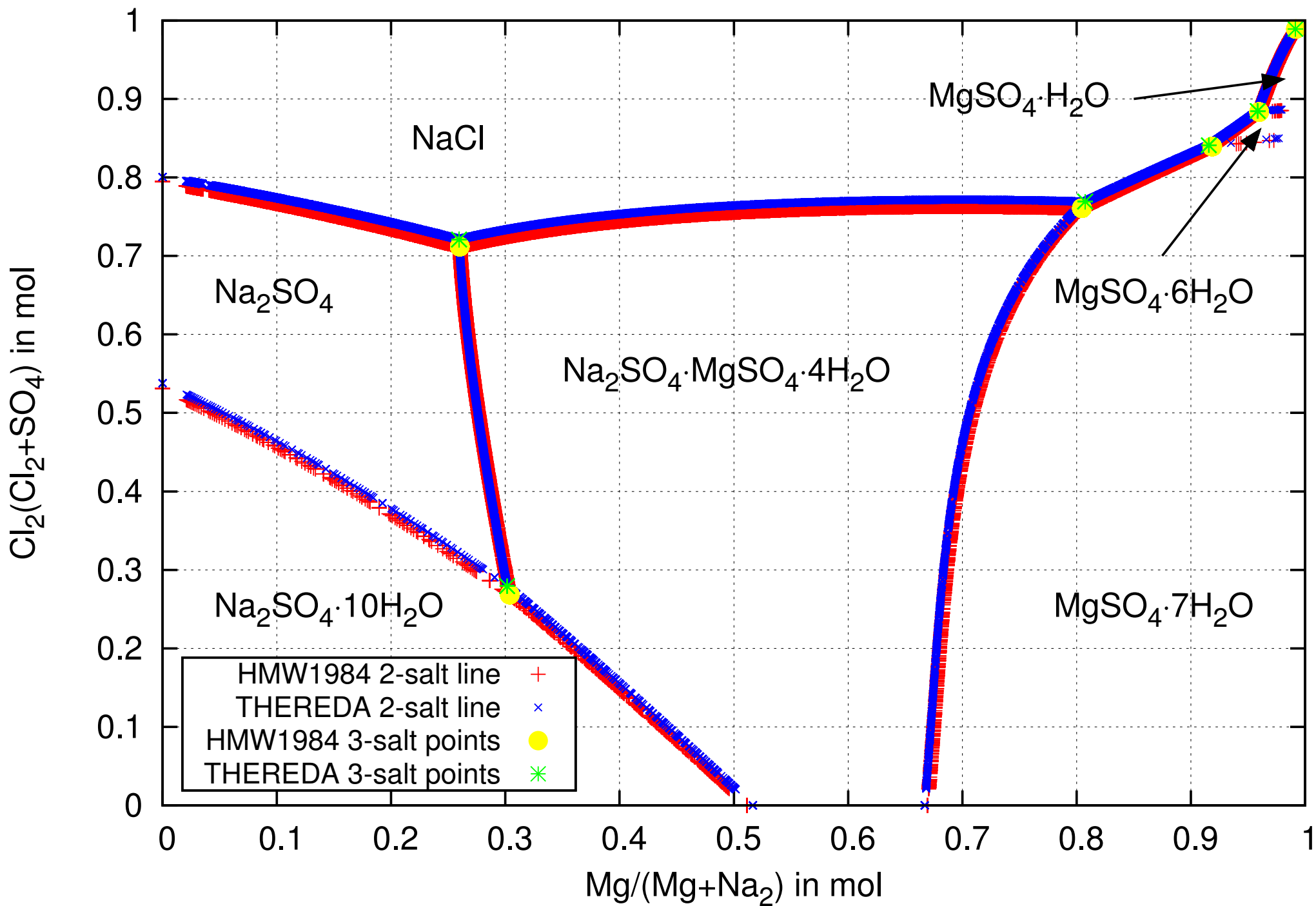
System \text{Na}^+, \text{Mg}^{++} // \text{Cl}^-, \text{SO}_4^{--} - \text{H}_2\text{O} at 298.15 K
