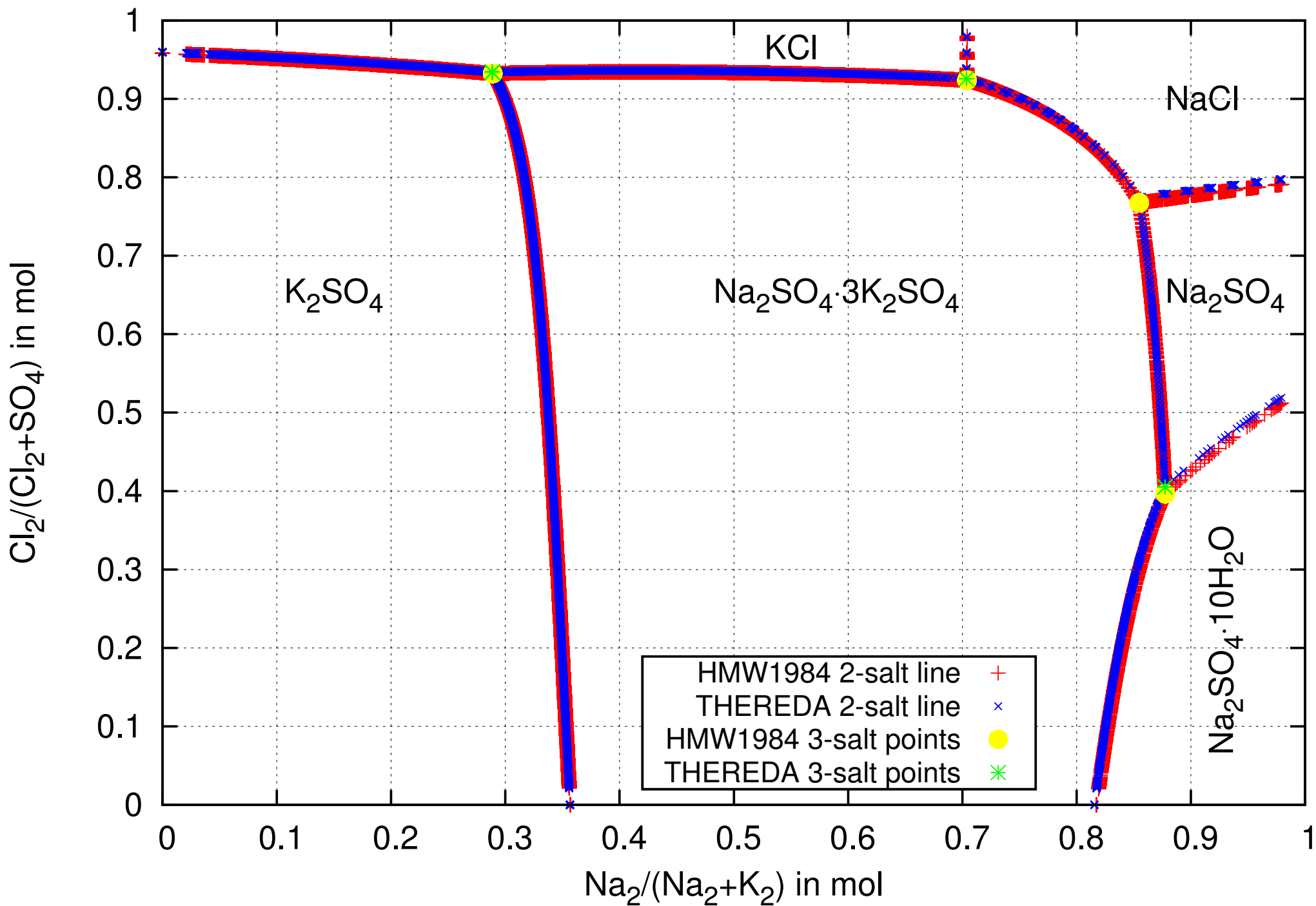
System \text{Na}^+, \text{K}^+ // \text{Cl}^-, \text{SO}_4^{2-} - \text{H}_2\text{O} at 298.15 K
