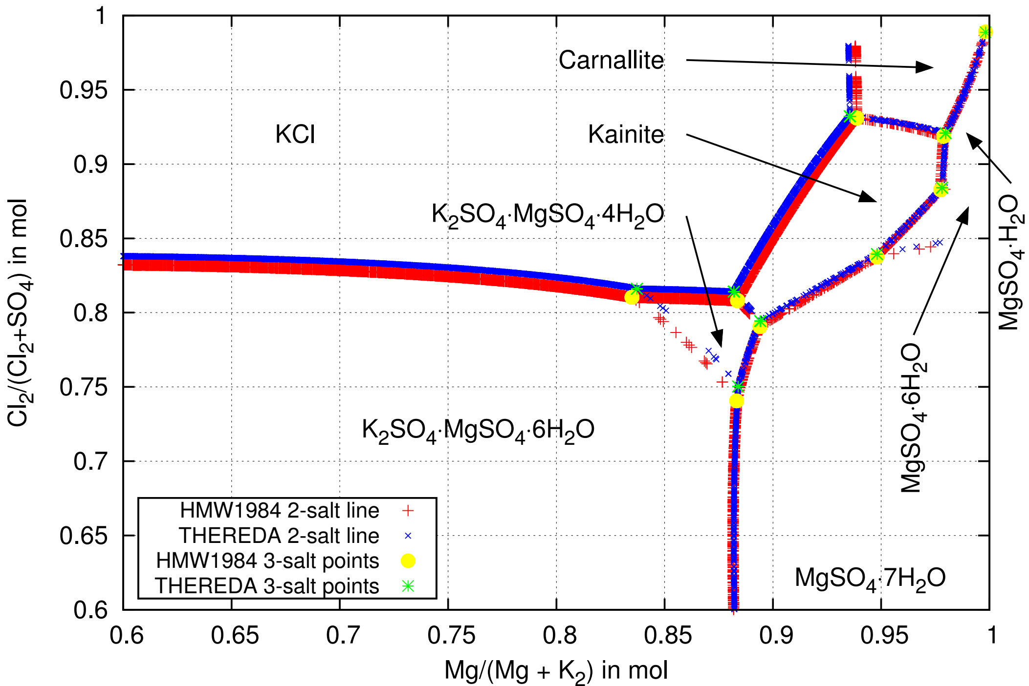
System \text{K}^+, \text{Mg}^{++} // \text{Cl}^-, \text{SO}_4^{--} - \text{H}_2\text{O} at 298.15 K
