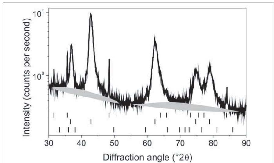
Abbildung 3: Diffraktogramm einer dünnen Schicht mit der chemischen Zusammensetzung \text{Ti}_{0,5}\text{Al}_{0,5}\text{N} . Breite Beugungslinien stammen vom kfz- \text{Ti}_{1-x}\text{Al}_x\text{N} , schmale Beugungslinien vom Wolframcarbid im Substrat. Graue Flächen markieren starke diffuse Streuung. Die Positionen der Beugungslinien von WC, \text{Ti}_{1-x}\text{Al}_x\text{N} und w-AlN (von oben nach unten) sind durch kleine Striche im unteren Teil des Bildes markiert.
