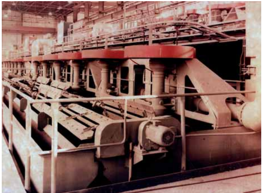
Bild 7: Flotationsanlage Zielitz
