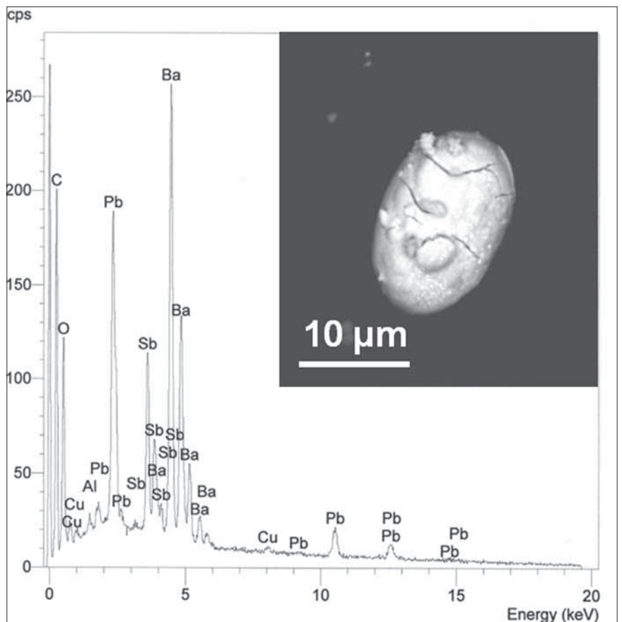
Abb. 3: Rasterelektronenmikroskopische Aufnahme und Röntgenemissionsspektrum eines Schmauchpartikels.
