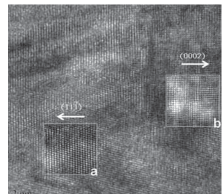
Abbildung 5: HRTEM-Aufnahme dünner Schicht, deren Diffraktogramm in Abb. 5 gezeigt wurde. Bereich (a) zeigt kfz- \text{Ti}_{1-x}\text{Al}_x\text{N} , Bereich (b) w-AlN.
