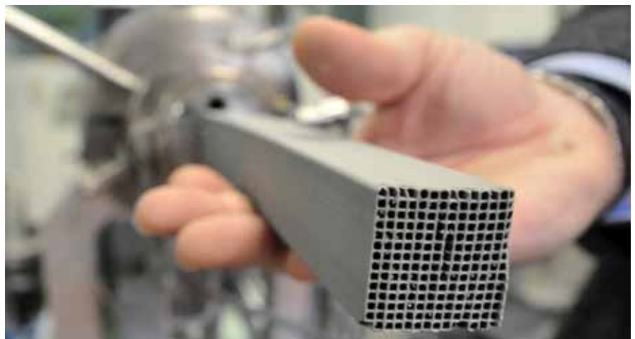
Wabenkörper auf der Basis eines austenitischen Stahlgusswerkstoffs und einer Keramik (10 Vol.% ZrO 2 )
