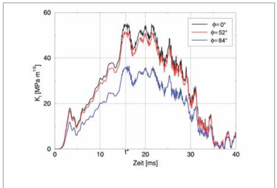
Bild 7: Berechneter zeitlicher Verlauf des Spannungsintensitätsfaktors
