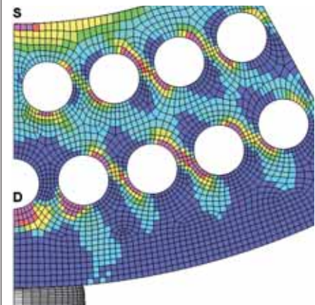
Bild 5: Verteilung der Hauptspannungen im Bereich oberhalb des Dorns
