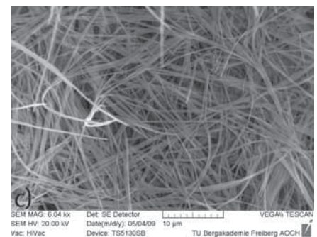
Abb. 5: Chemisch langzeitstabile Bindemittelphase 3 \text{ Mg(OH)}_2 \cdot \text{MgCl}_2 \cdot 8 \text{ H}_2\text{O} (3-1-8) des MgO-Baustoffs für Anwendung im Kalisalz: a) REM-Bild der Kristallite nach dem Abbinden (neue Rezeptur); b) Aufbau der Kristallstruktur; c) REM-Bild der Kristallite in Gegenwart von Gleichgewichts-Salzlösung
