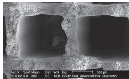
Bild 2: Wabenkörper Versatz Z10, REM-Aufnahme
