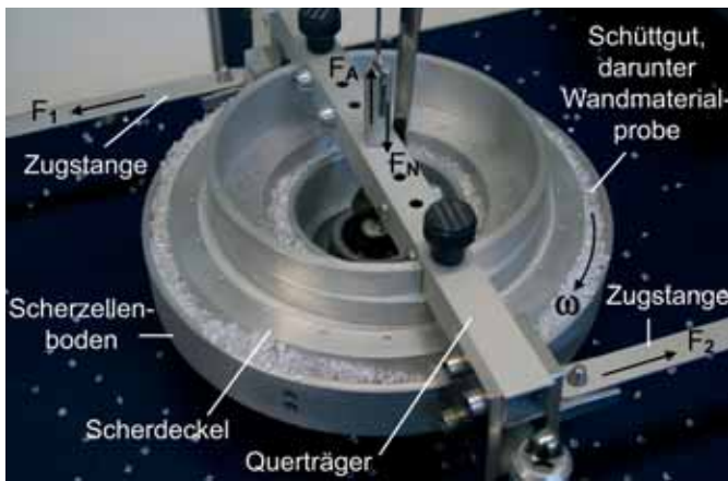
Abbildung 1: Schulze-Ringscherzelle, gefüllt mit PET-Granulat
