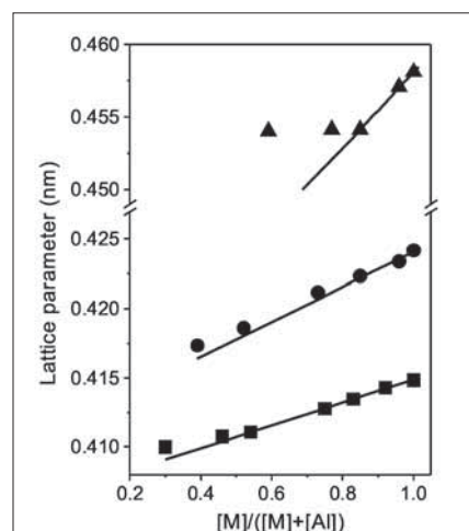
Abbildung 4: Abhängigkeit des spannungsfreien Gitterparameters in nanokristallinen \text{Zr}_{1-x}\text{Al}_x\text{N} ( \blacktriangle ), \text{Ti}_{1-x}\text{Al}_x\text{N} ( \bullet ) und \text{Cr}_{1-x}\text{Al}_x\text{N} ( \blacksquare ) Dünnschicht-Nanokompositen vom gesamten Aluminiumgehalt in den Schichten. Grau markierte Bereiche bezeichnen die zweiphasigen Proben.
