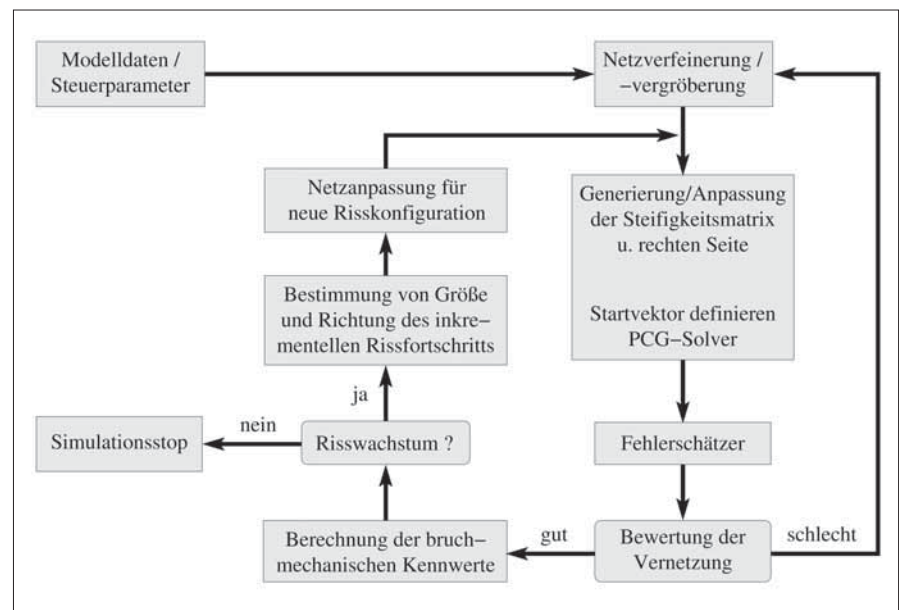
Bild 1: Programmablaufschema (PCG: Preconditioned Conjugate Gradient)
