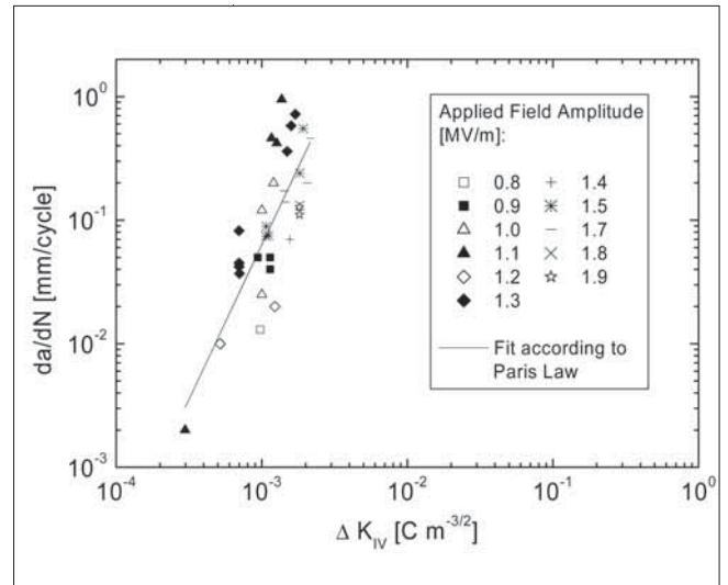
Bild 11: Risswachstumsrate als Funktion des zyklischen Feldintensitätsfaktors
