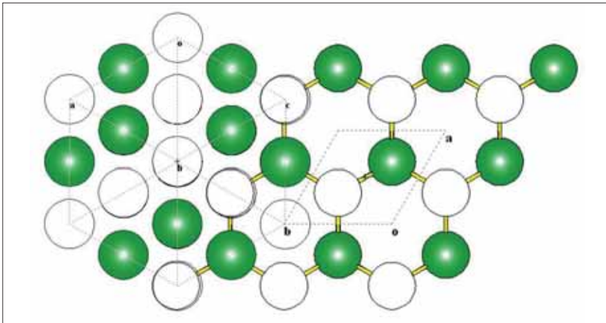
Abbildung 6: Atomares Modell der Grenzfläche zwischen kfz-Ti 1-x Al x N (links) und w-AlN (rechts) in einem (Ti,Al)N-Nanokomposit entsprechend der kristallographischen Orientierung aus Abb. 5.
