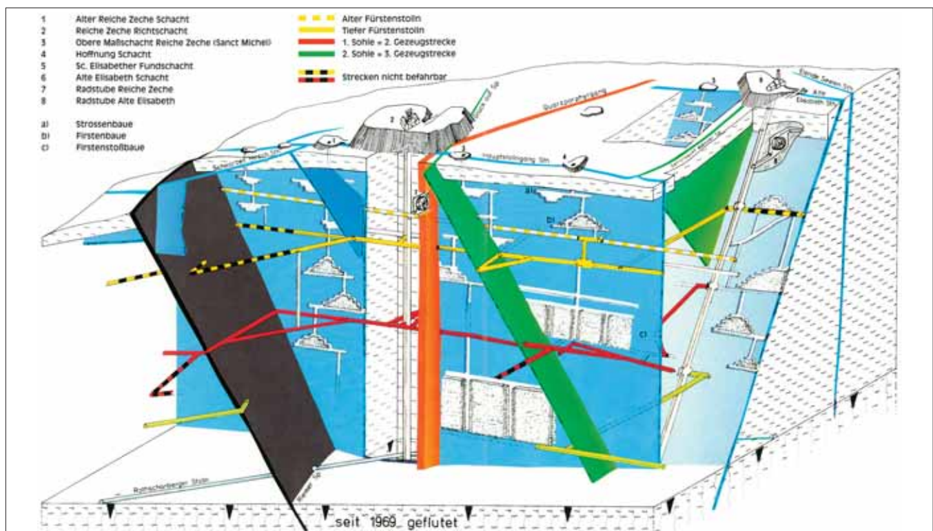
Blockbild des Lehrbergwerks. Zeichnung: Bayer/Meyer
