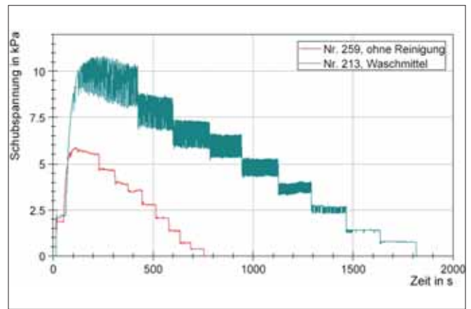
Abbildung 2: Vergleich der Schubspannungen bei ungereinigtem und gereinigtem Wandmaterial bei verschiedenen Auflasten zwischen 28 kPa und 2 kPa
