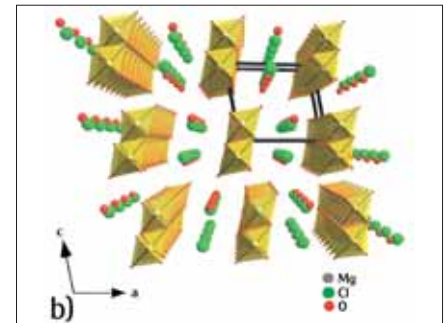
Abb. 4: Bindemittelphase 5 \text{ Mg(OH)}_2 \cdot \text{MgCl}_2 \cdot 8 \text{ H}_2\text{O} (5-1-8) des MgO-Baustoffs a) REM-Bild der fein verfilzten Kristallite im Baustoffprobekörper; b) Aufbau der Kristallstruktur
