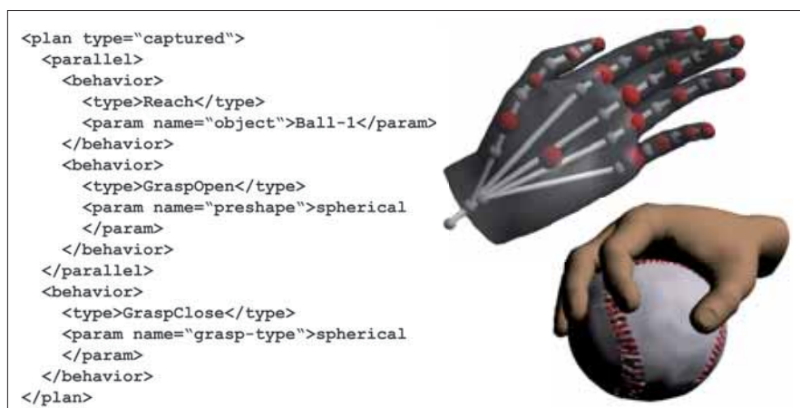
Abbildung 4: Links: Aus Benutzerinteraktion generierter Plan zum Greifen eines Balls. Rechts: Das virtuelle Handmodell ist mit kugelförmigen Kollisionssensoren ausgestattet; beim Zugreifen (Behavior Grasp-Close) werden die Finger solange geschlossen, bis eine Kollision mit dem Zielobjekt auftritt.
