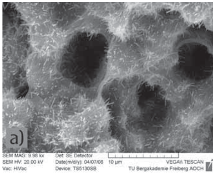
Abb. 4: Bindemittelphase 5 \text{ Mg(OH)}_2 \cdot \text{MgCl}_2 \cdot 8 \text{ H}_2\text{O} (5-1-8) des MgO-Baustoffs a) REM-Bild der fein verfilzten Kristallite im Baustoffprobekörper; b) Aufbau der Kristallstruktur
