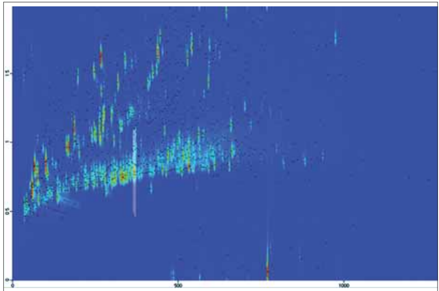
Abb. 5: 2D-Gaschromatogramm für flüchtige organische Verbindungen aus einer Patronenhülse.
