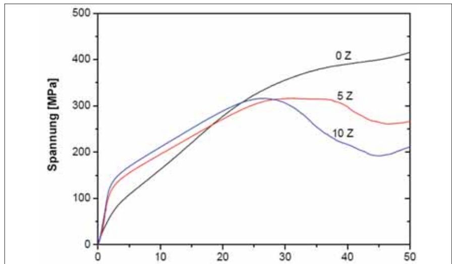
Bild 7: Druckversuch, Spannungs-Stauchungs-Diagramm
