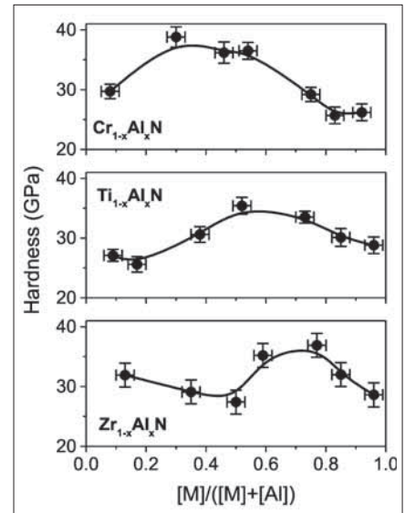
Abbildung 7: Änderung der Härte von nanokristallinen (Cr,Al)N-, (Ti,Al)N- und (Zr,Al)N-Dünnschicht-Nanokompositen mit unterschiedlichem Aluminiumgehalt.
