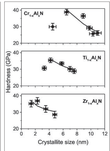
Abbildung 2: Änderung der Härte in nanokristallinen (Cr,Al)N-, (Ti,Al)N- und (Zr,Al)N-Dünnschicht-Nanokompositen mit abnehmender Kristallitgröße. Die Linie zeigt den Härteanstieg nach Hall [7] und Petch [8], der nach Gl. (1) an die Messdaten (bei steigender Härte) angepasst wurde.
