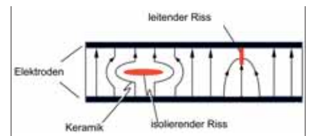
Bild 8: Versagen piezoelektrischer Bauelemente infolge elektrischer Felder an Defekten
