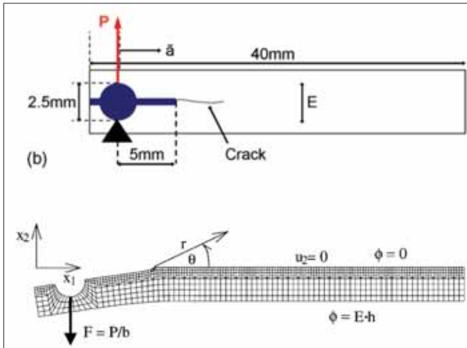
Bild 10: DCB-Probe für zyklische elektrische Felder E mit mechanischer Vorlast P (links) und verformtes FEM-Netz (rechts)
