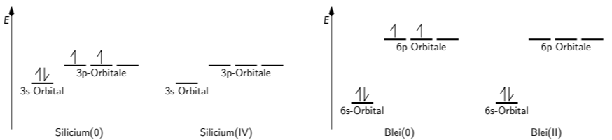
Abb.2: Energieschema der s- und p-Orbitale bei Si und Pb.
